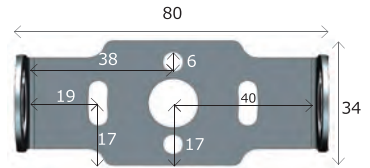
・カメラ設置ブラケット寸法(mm)
