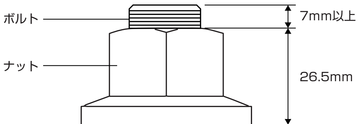
適合ボルトナット (装着できるボルトナット)
